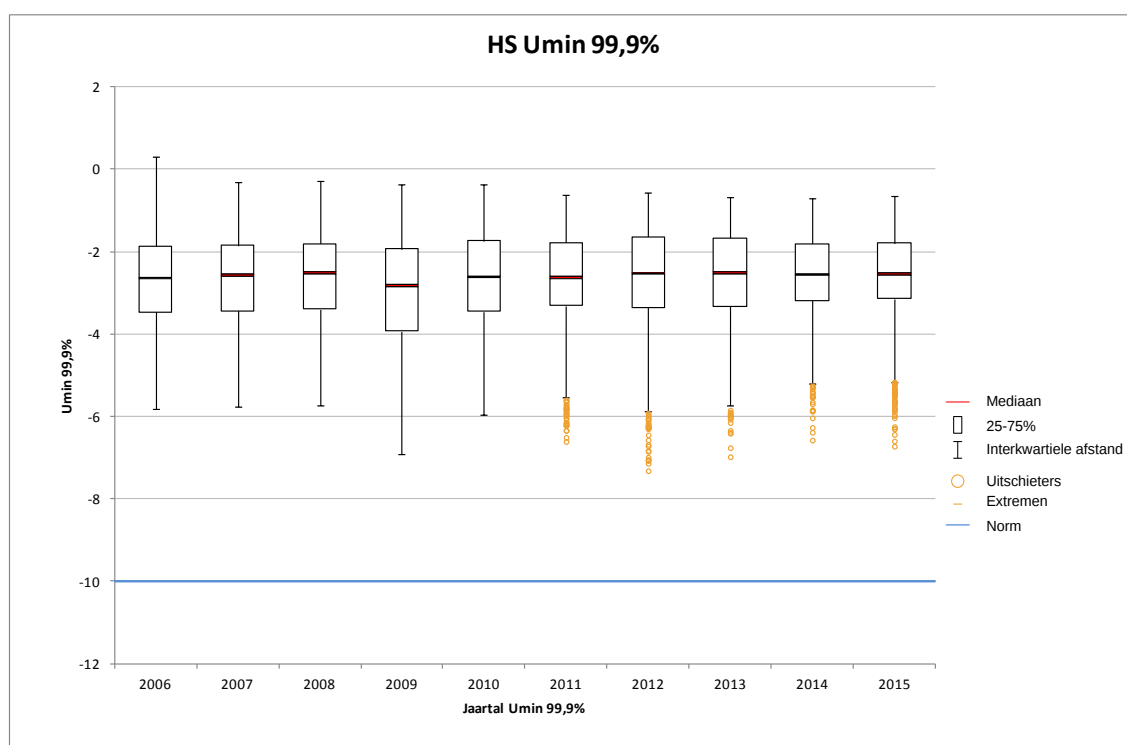
Figuur 4.6: Langzame spanningsvariatie (Umin) HS-netvlak, 2006-2015
