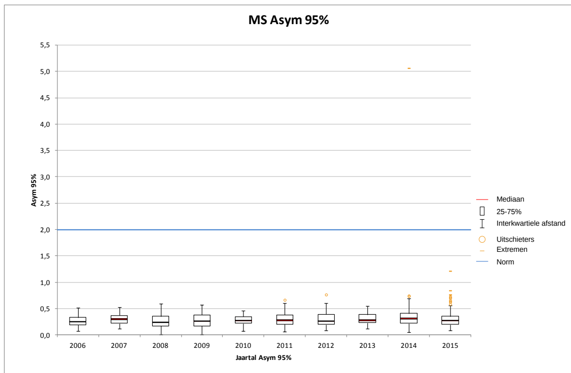
Figuur 4.14: Spanningsasymmetrie MS-netvlak, 2006-2015
