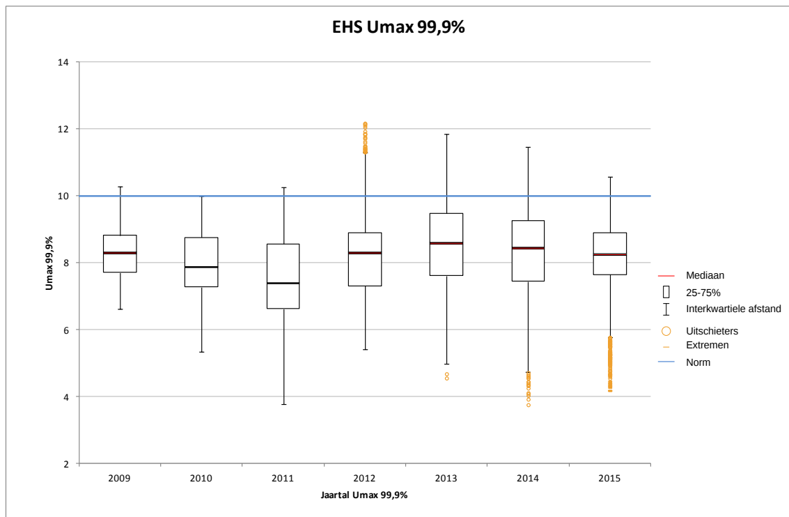
Figuur 4.7: Langzame spanningsvariatie ( U_{max} ) EHS-netvlak, 2009-2015
