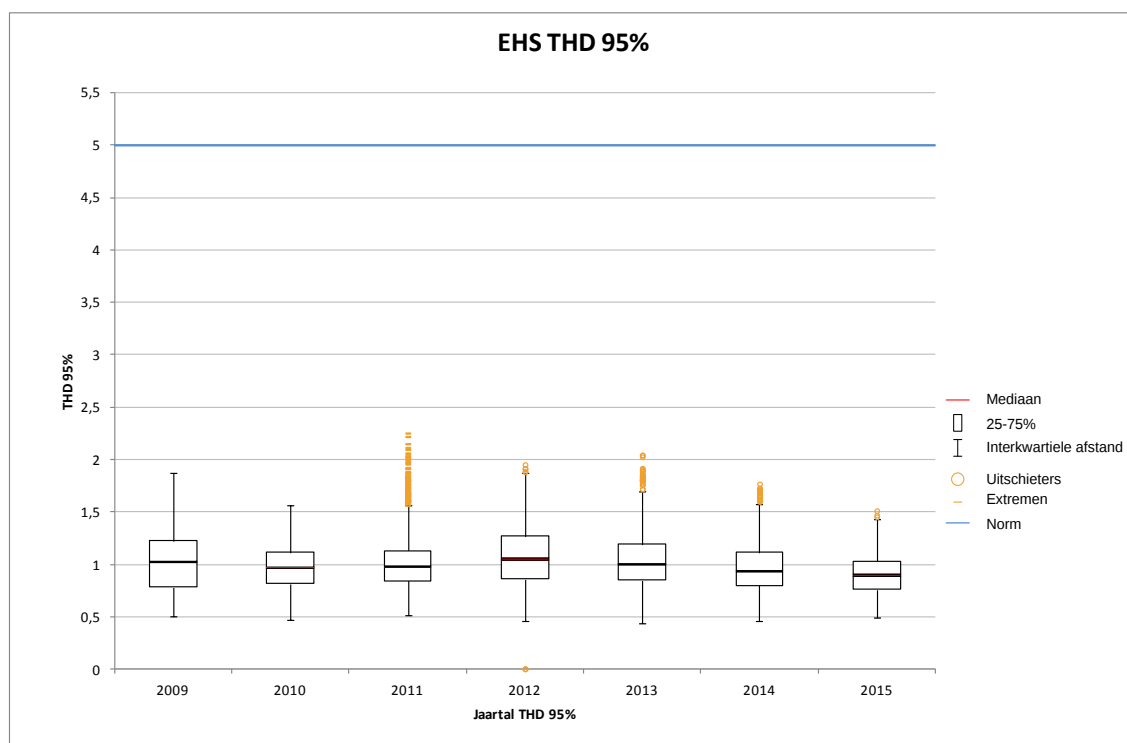
Figuur 4.20: Totale harmonische vervorming EHS-netvlak, 2009-2015
