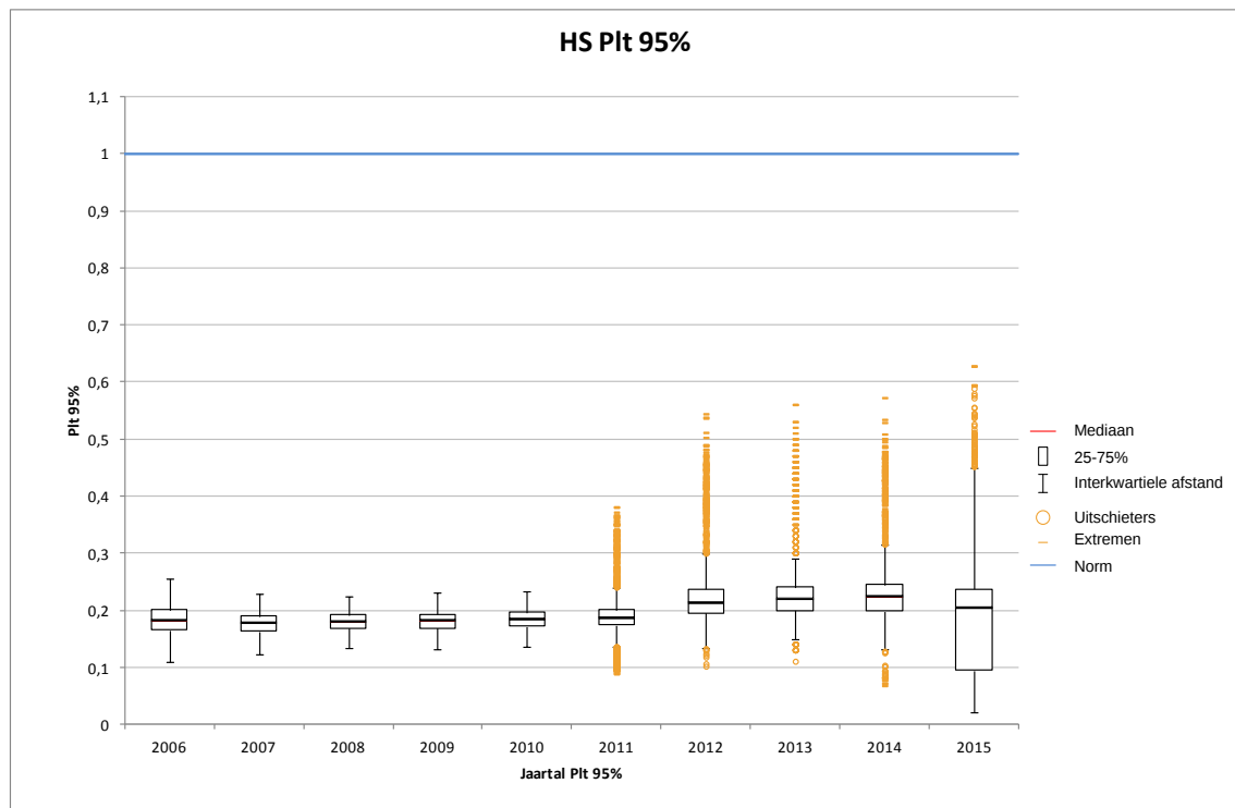
Figuur 4.11: Snelle spanningsvariatie HS-netvlak, 2006-2015
