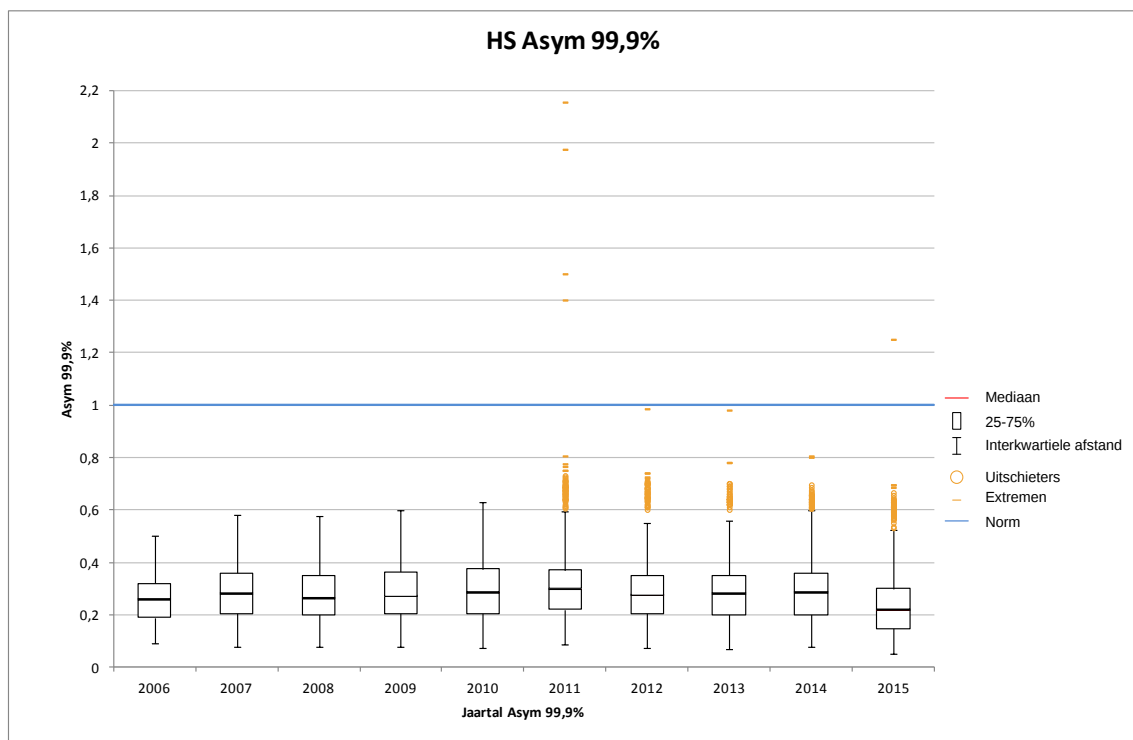
Figuur 4.15: Spanningsasymmetrie HS-netvlak, 2006-2015
