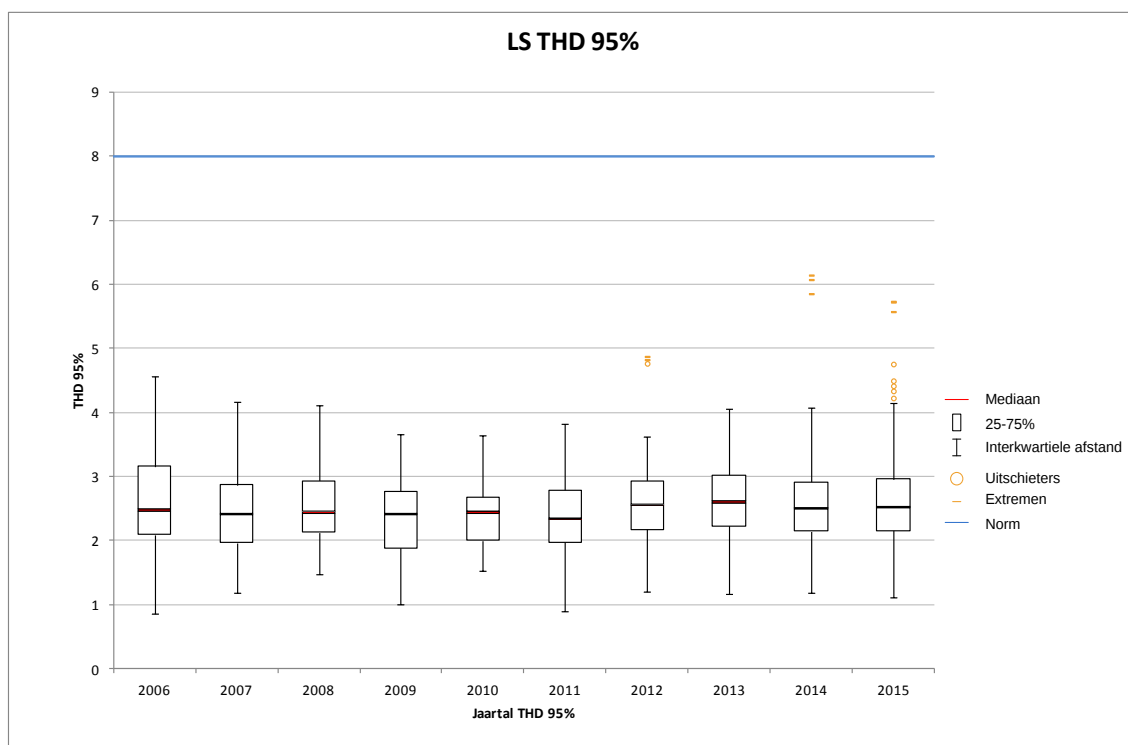
Figuur 4.17: Totale harmonische vervorming LS-netvlak, 2006-2015
