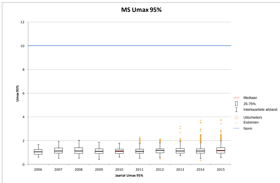
Figuur 4.3: Langzame spanningsvariatie ( U_{max} ) MS-netvlak, 2006-2015
