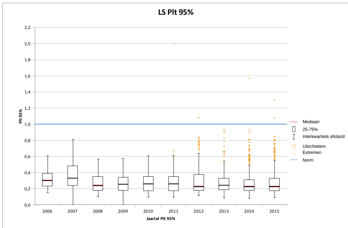
Figuur 4.9: Snelle spanningsvariatie LS-netvlak, 2006-2015
