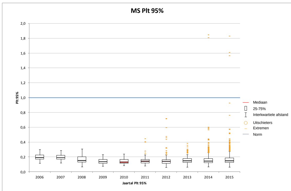
Figuur 4.10: Snelle spanningsvariatie MS-netvlak, 2006-2015
