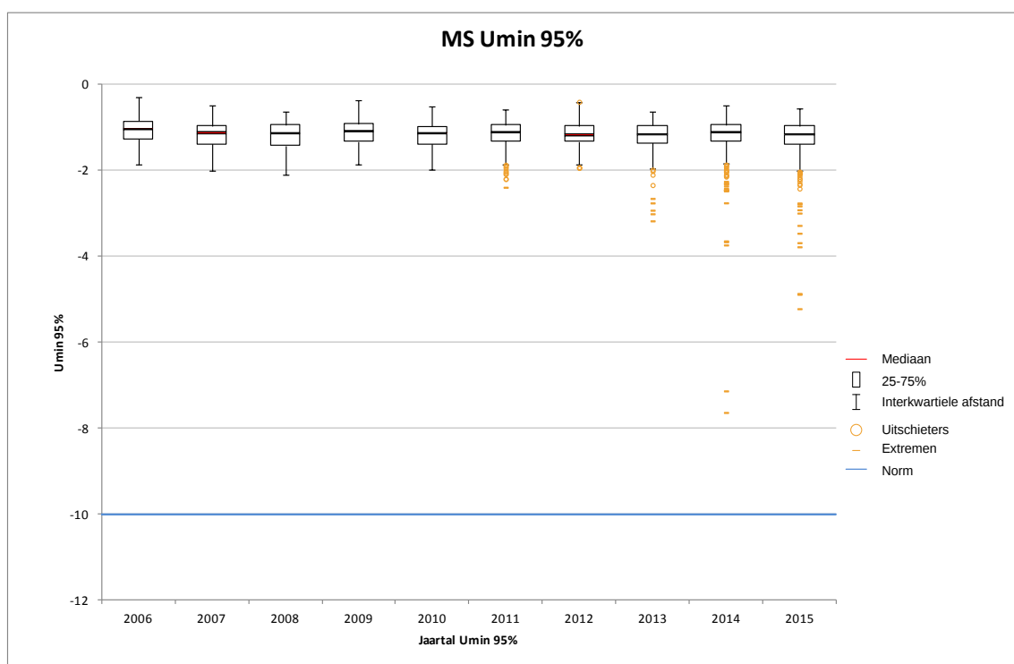
Figuur 4.4: Langzame spanningsvariatie ( U_{min} ) MS-netvlak, 2006-2015
