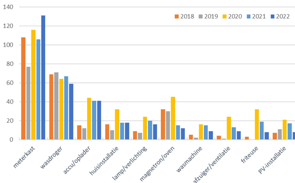
Figuur 3.4: top 10 van het aantal ongevallen per apparaat/installatie, 2018-2022
