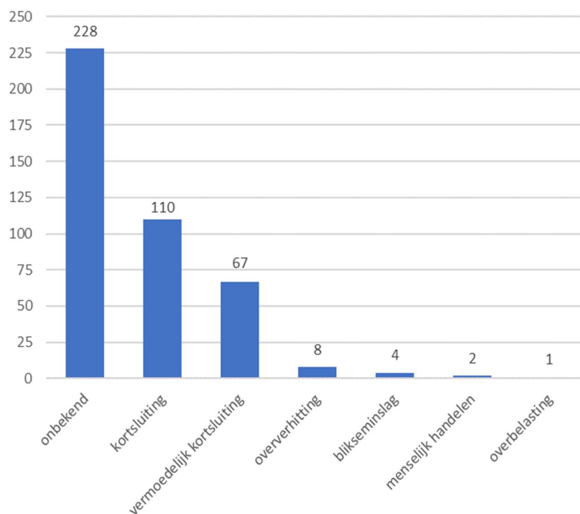
Figuur 2.4: oorzaken van ongevallen, 2022
