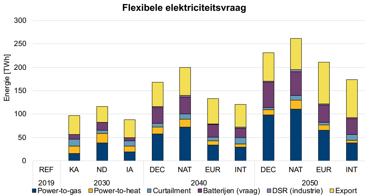
Figuur 30. Overzicht flexibele vraag voor overschotten in TWh.
