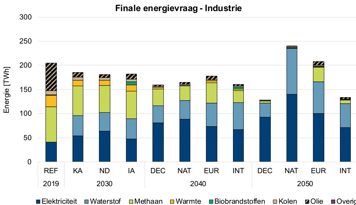
Figuur 60. Finale energie vraag – industrie (energetisch). De productie van SAF is niet gemodelleerd in het ETM en de bijbehorende energievraag is niet opgenomen in deze figuur.
