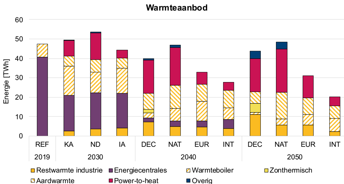
Figuur 17. Aanbod van warmte in 2019 en ontwikkeling tot 2050, in TWh.
