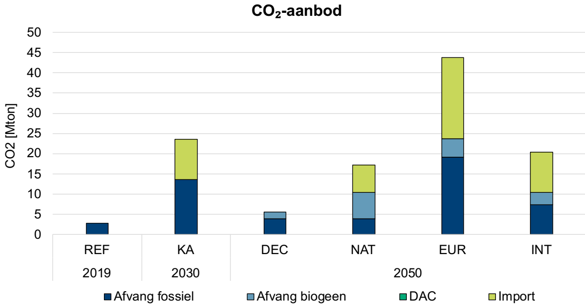
Figuur 45 - CO 2 balans (aanbod aan koolstof). DAC wordt in de basis scenario's van II3050 niet ingezet.
