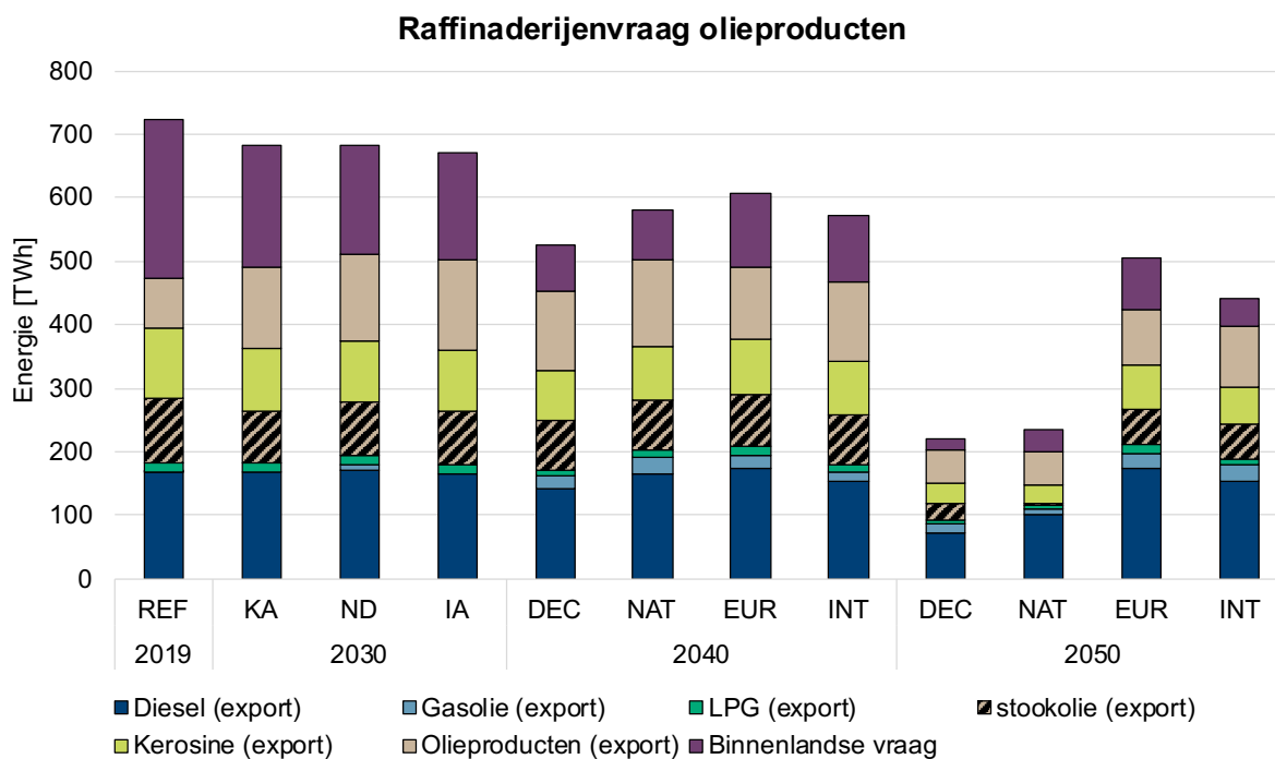
Figuur 66 - Finale vraag van raffinaderijen naar olie producten
