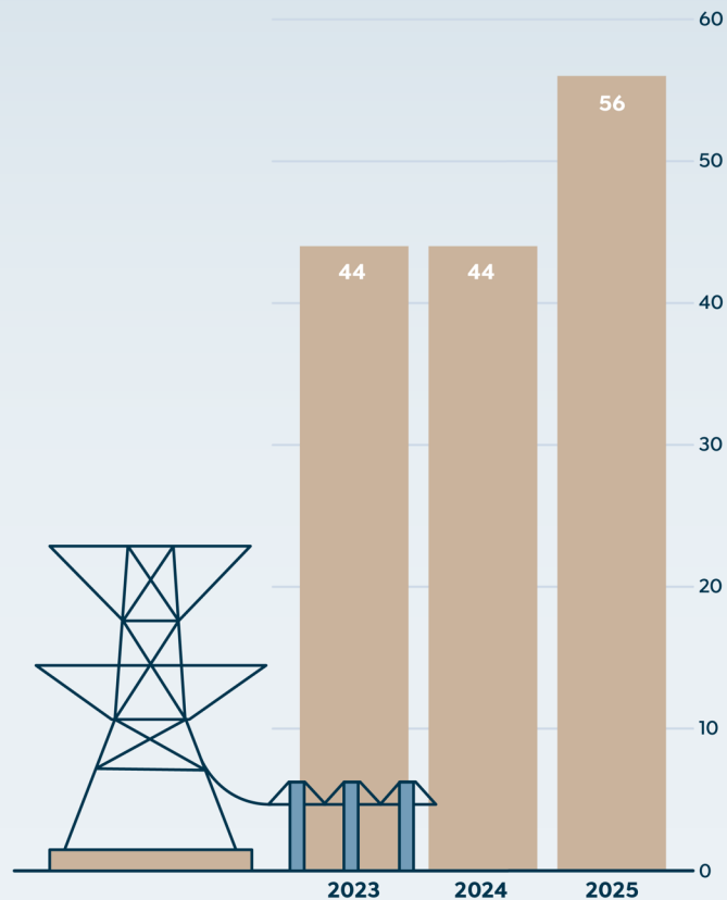
Gerealiseerde HS-netten
