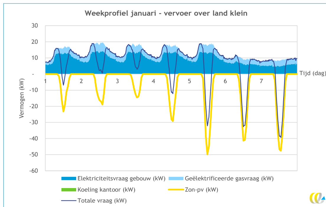
Figuur 70 - Elektriciteitsvraag en -opwek van het gebouw week 1 van januari
