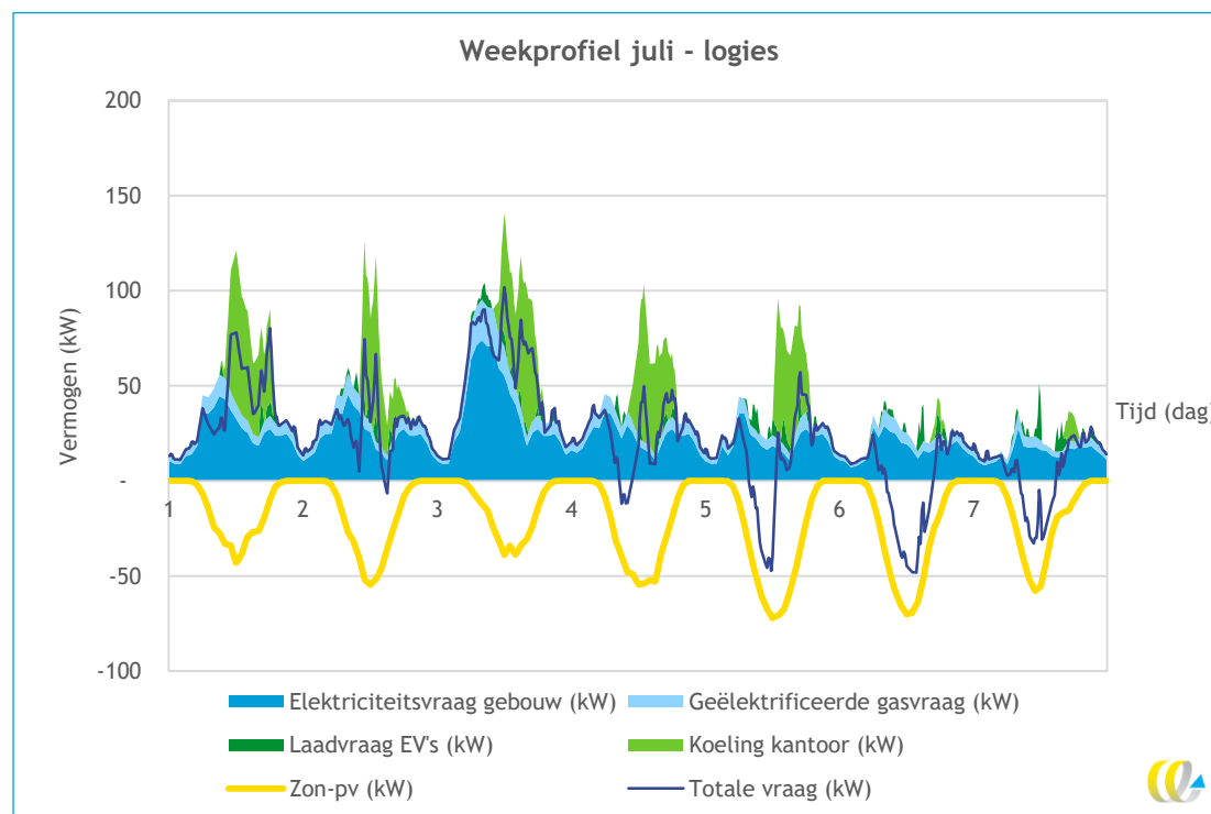
Figuur 62 - Elektriciteitsvraag van de casus logies voor de eerste week van juli
