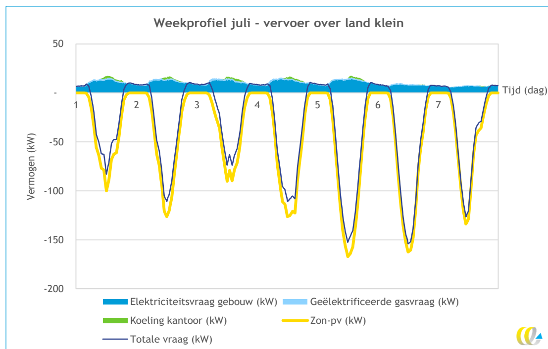
Figuur 71 - Elektriciteitsvraag en -opwek van het gebouw week 1 van juli
