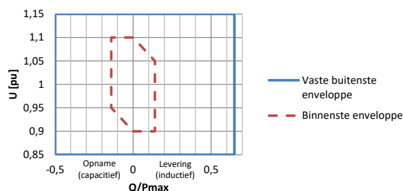
U-Q/Pmax-profiel van een DC-aangesloten PPM (Unom < 300kV)
